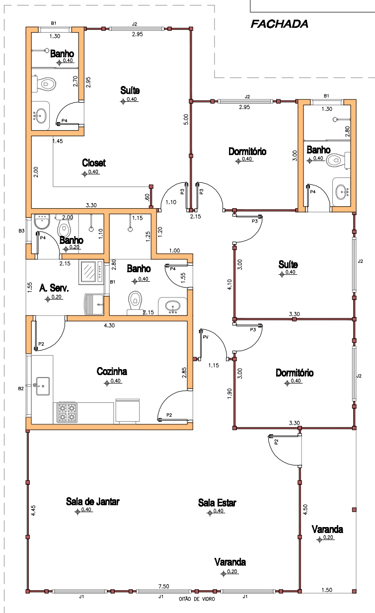
PLANTA BAIXA
