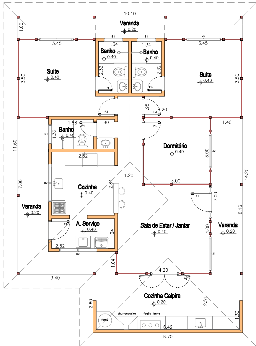
PLANTA BAIXA
