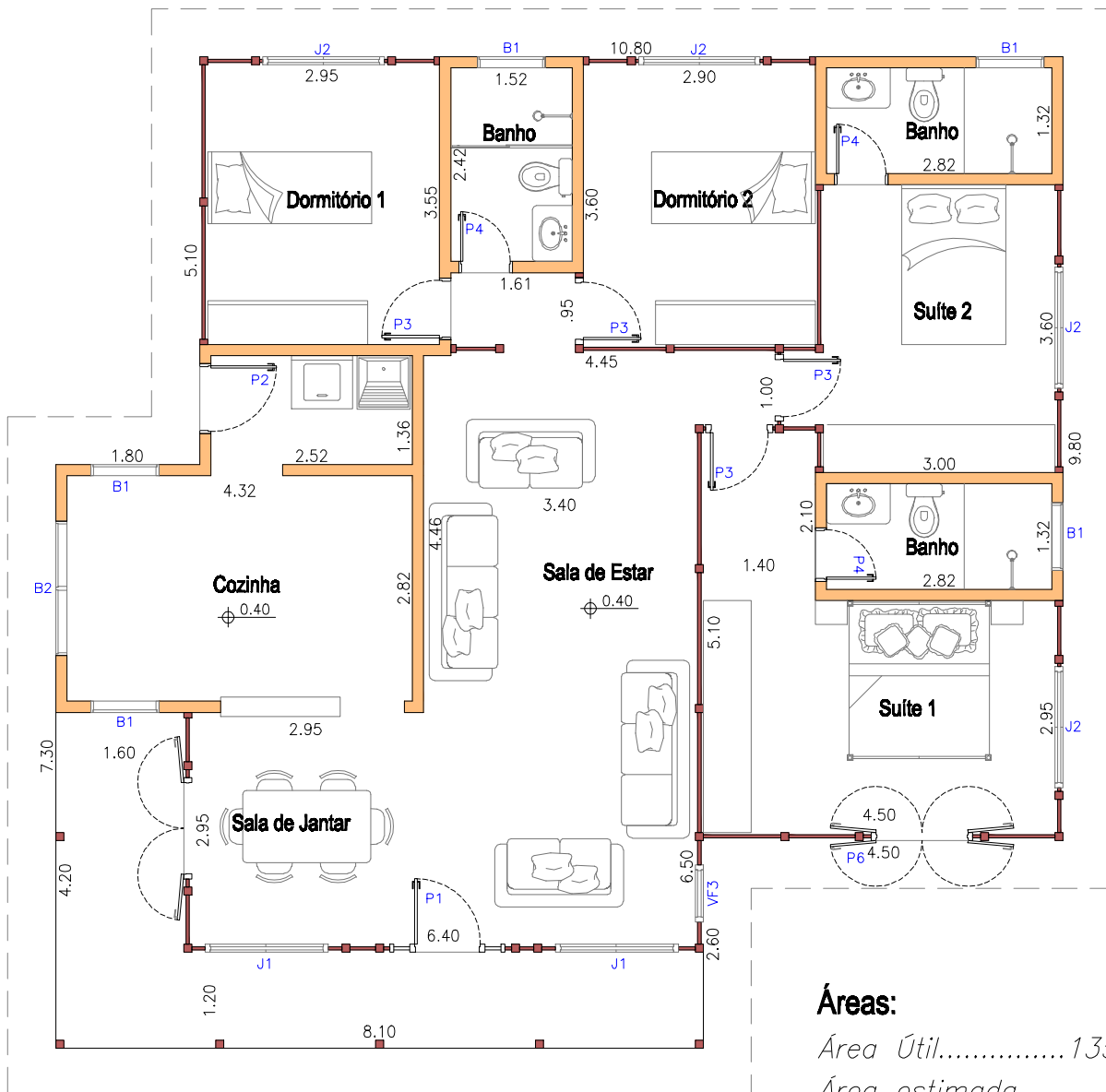
PLANTA BAIXA
